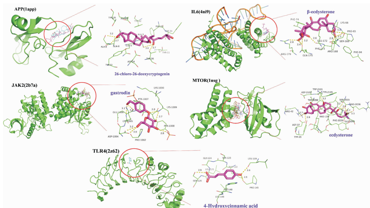
图 4 关键靶点与其对应成分的分子对接结合模式图
